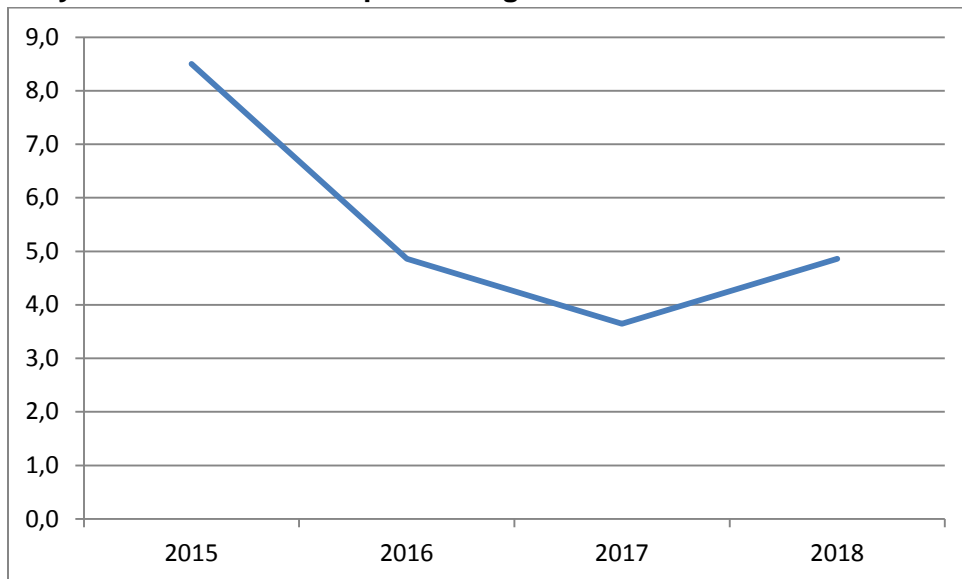
Figura 1. Comportamiento de tasas de incidencia de Mortalidad por IRA 2015, 2016, 2017 y 2018 a semana 18 epidemiológica
